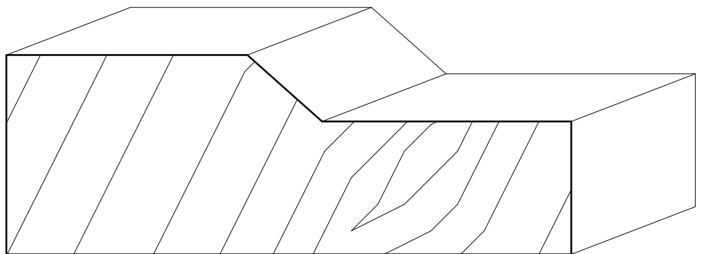
PL-123 1 1/2" X 4 1/4"
