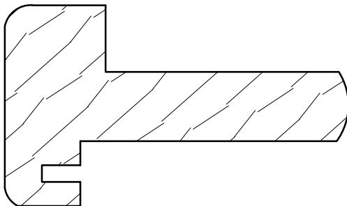
T-AST-4 1 \frac{1}{2}'' \times 2 \frac{9}{16}'' FOR 1 \frac{3}{4}'' DOOR
