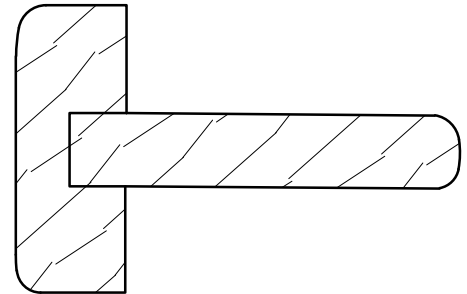
T-AST-5 1 \frac{1}{2}'' \times 2 \frac{5}{16}'' FOR 1 \frac{3}{4}'' DOOR
