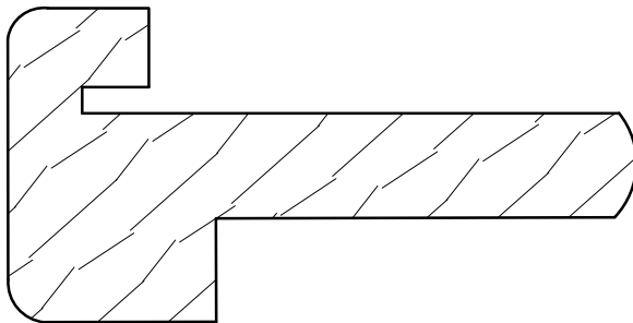
T-AST-3 1 \frac{1}{2}'' \times 3'' FOR 1 \frac{3}{4}'' DOOR
