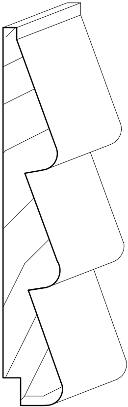
FL-12 \frac{5}{8}'' \times 4''
